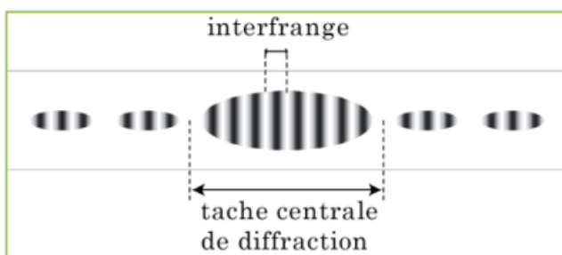
Figure obtenue avec des fentes d'Young
