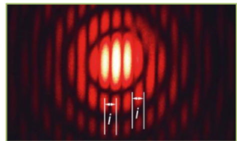
Figure obtenue avec des trous d'Young
